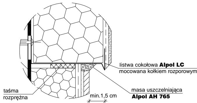
szczegół A
